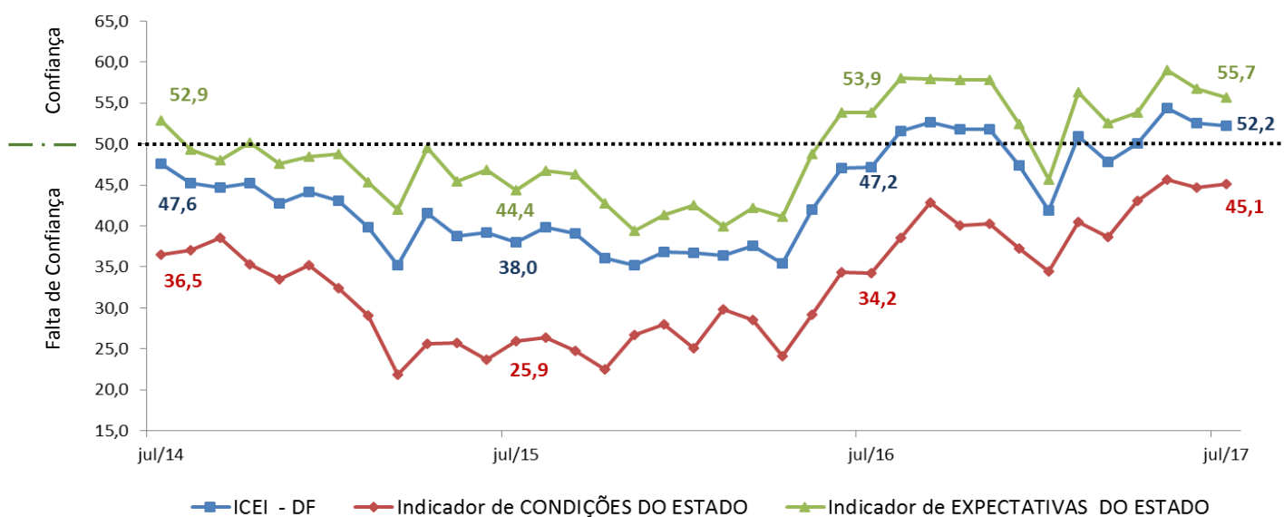
Gráfico 2: ICEI/DF (índices)
